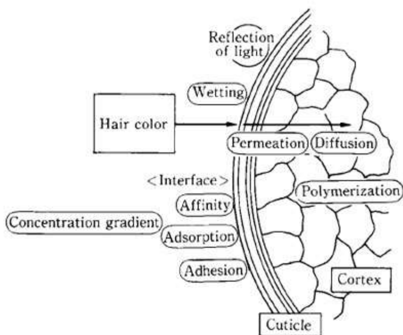
شکل: دیاگرام فرآیندهای فیزیکی و شیمیایی درگیر در پروسه رنگ شدن موها
